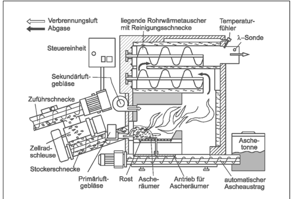
Abb. 16: Funktionsschema einer 50 kW-Holz hackschnitzelfeuerung
