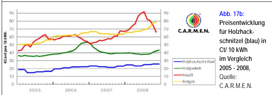
Abb. 17: Holzhackschnitzelheizungen: jährliche Bestände 2000 - 2007, Preisentwicklung im Vergleich
