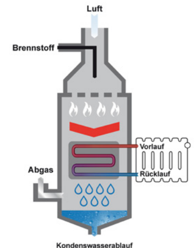
01 Funktionsweise Brennwerttechnik
